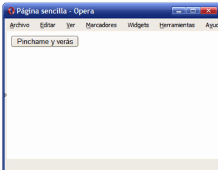
Figura 6.1. Página HTML
