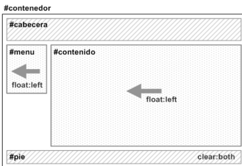
Figura 12.8. Propiedades CSS necesarias en el diseño a dos columnas con cabecera y pie de página
